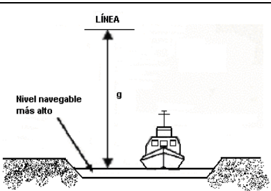
Figura 13. 4. Distancia “f” y “g” para cruces con ferrocarriles y ríos
